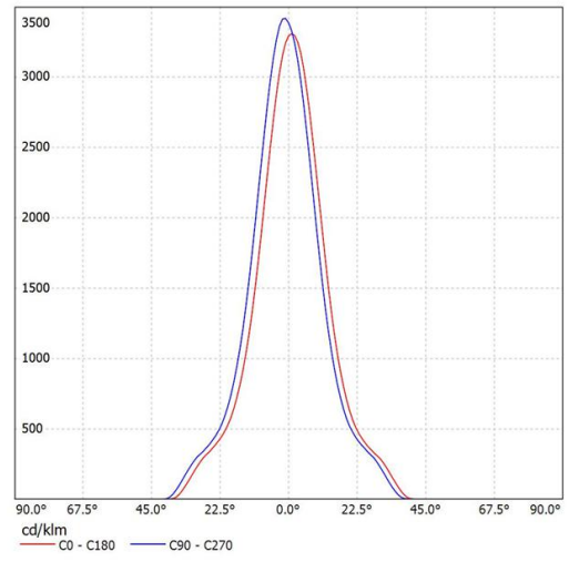
SL-05024A K:4.35cd/lm,LED:1507
