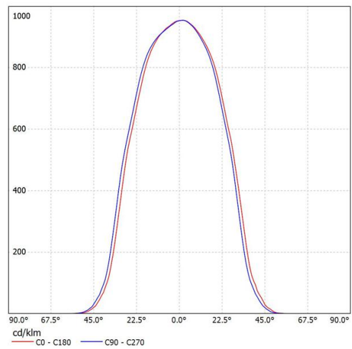
SL-05060A K:1.24cd/lm,LED:1507
