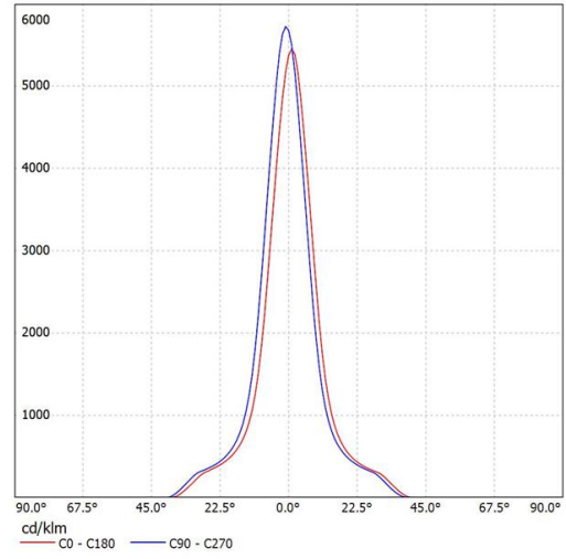
SL-05015A K:7.35cd/lm,LED:1507
