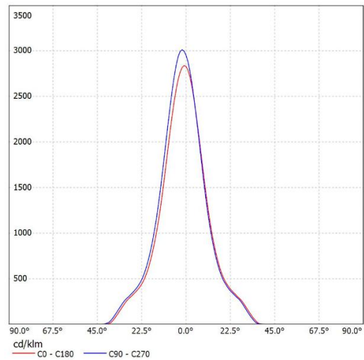
SL-05024A K:4.33cd/lm,LED:CXM-9
